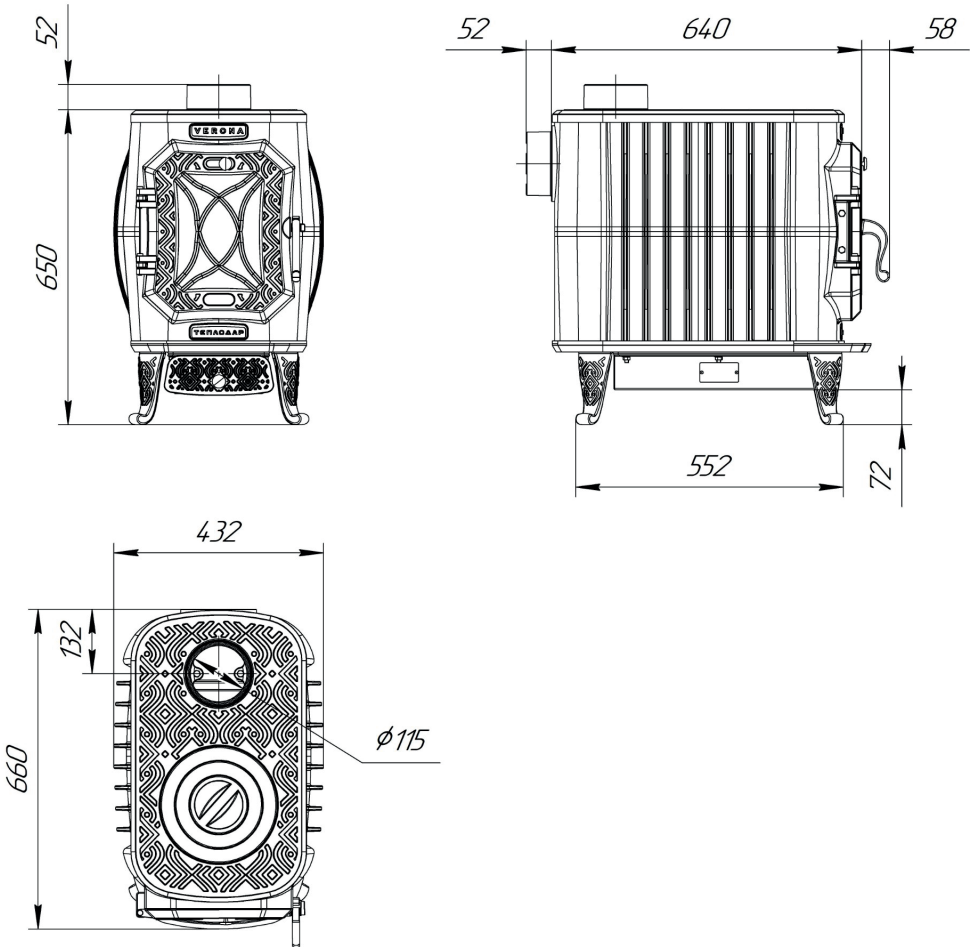
Печь VERONA-200
